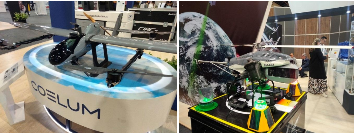
A la izquierda el ART Coelum desarrollado por la Corporación de la Industria Aeronáutica Colombiana, CIAC, y que ha superado las más exigentes pruebas. Esta disponible para el mercado nacional y de exportación. A la derecha, un drone "Frankenstein", en que se unieron exitosamente un viejo ART tipo helicóptero que había sido dado de baja por la Fuerza Aeroespacial Colombiana, con la cabeza de un ART tipo Scan Eagle en igual condición. Creando así un drone completamente funcional que integra los sensores de alta tecnología del San Eagle en una plataforma con capacidad para el despegue y aterrizaje vertical. Eso lo hizo la gente de ciencia y tecnología de la FAC, un equipo liderado por un Jefe Técnico retirado. Ahí en la mesa hay otras cosas también muy interesantes. Expodefensa 2023, Bogotá.
